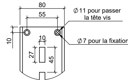
DÉTAIL A ECHELLE 1 : 4
